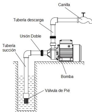
A Ejemplo de Instalación CORRECTA
