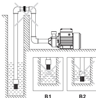
B Ejemplos de Instalaciones INCORRECTAS
